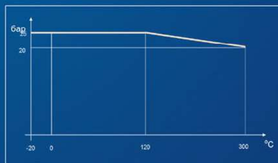
График: Зависимость давление-температура
